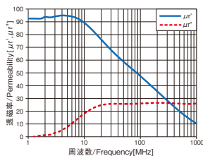
MG-12シリーズ/MG-12 Series
