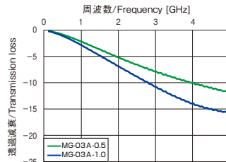
MG-03Aシリーズ/MG-03A Series
