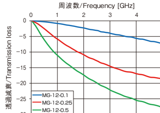
MG-12シリーズ/MG-12 Series
